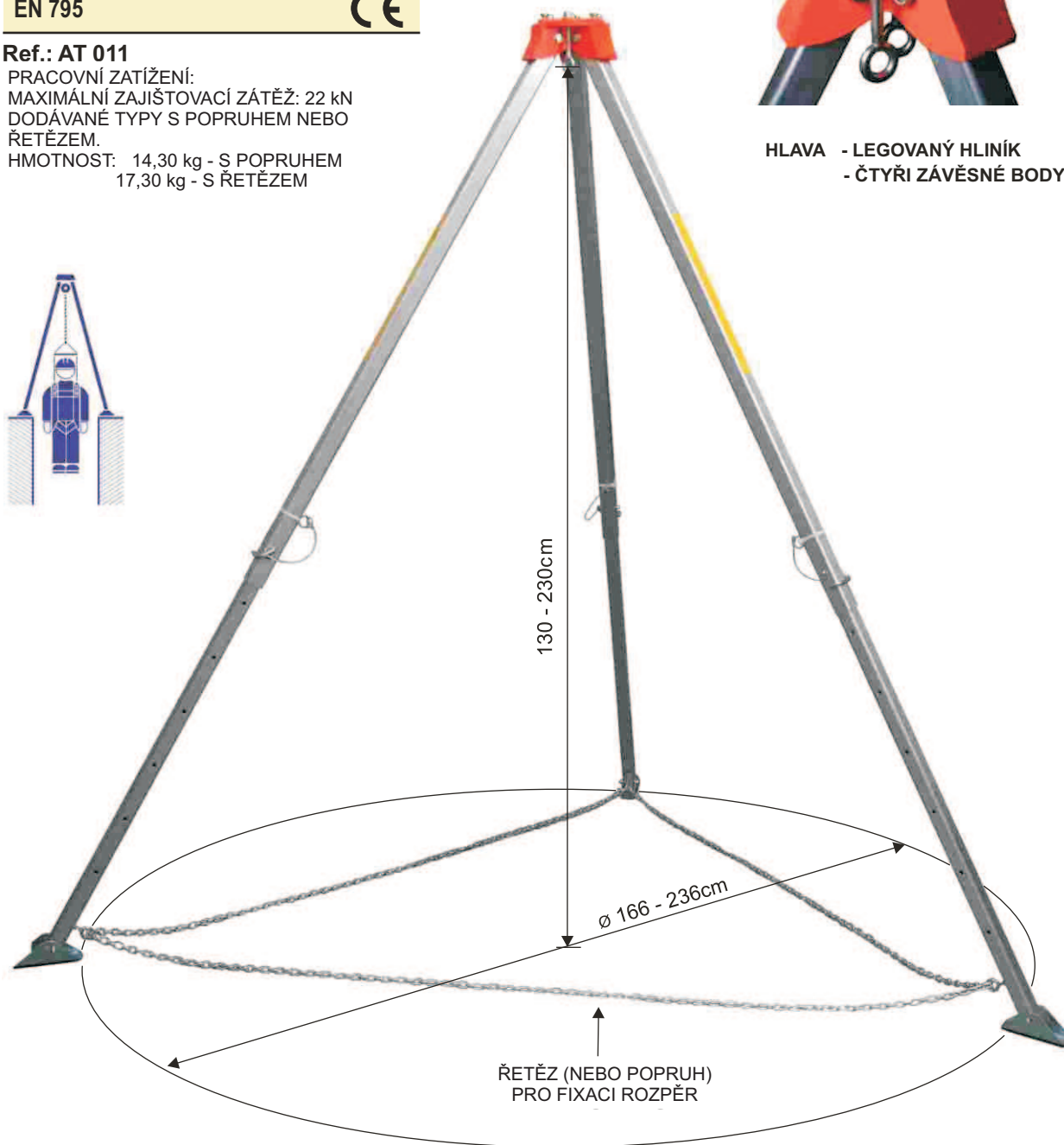
ROZMĚRY TROJNOŽKY
